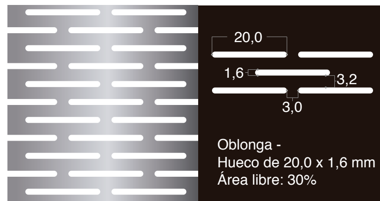
Dimensión: 1.22 x 2.44 mts Calibre: 18 Material: Acero CR
